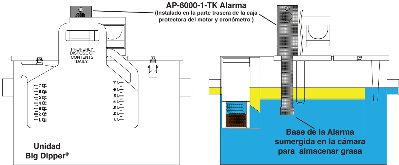
Vista Lateral
